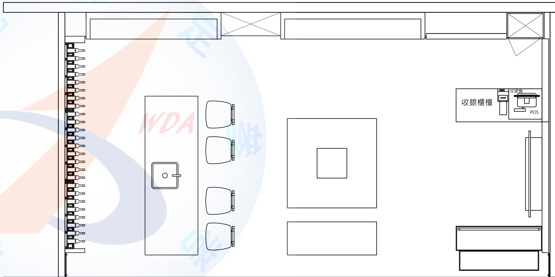
平面配置圖
