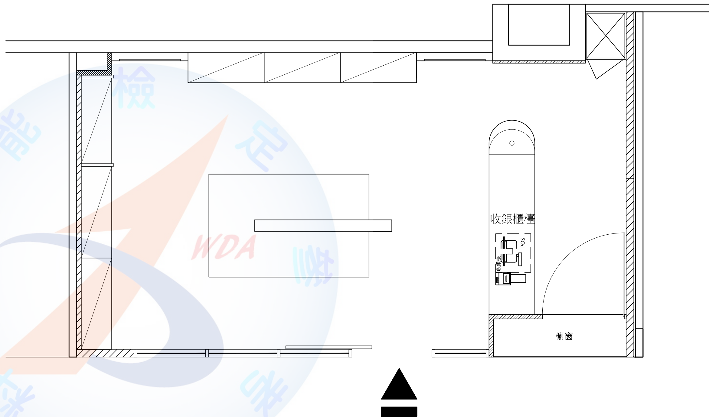
平面配置圖
