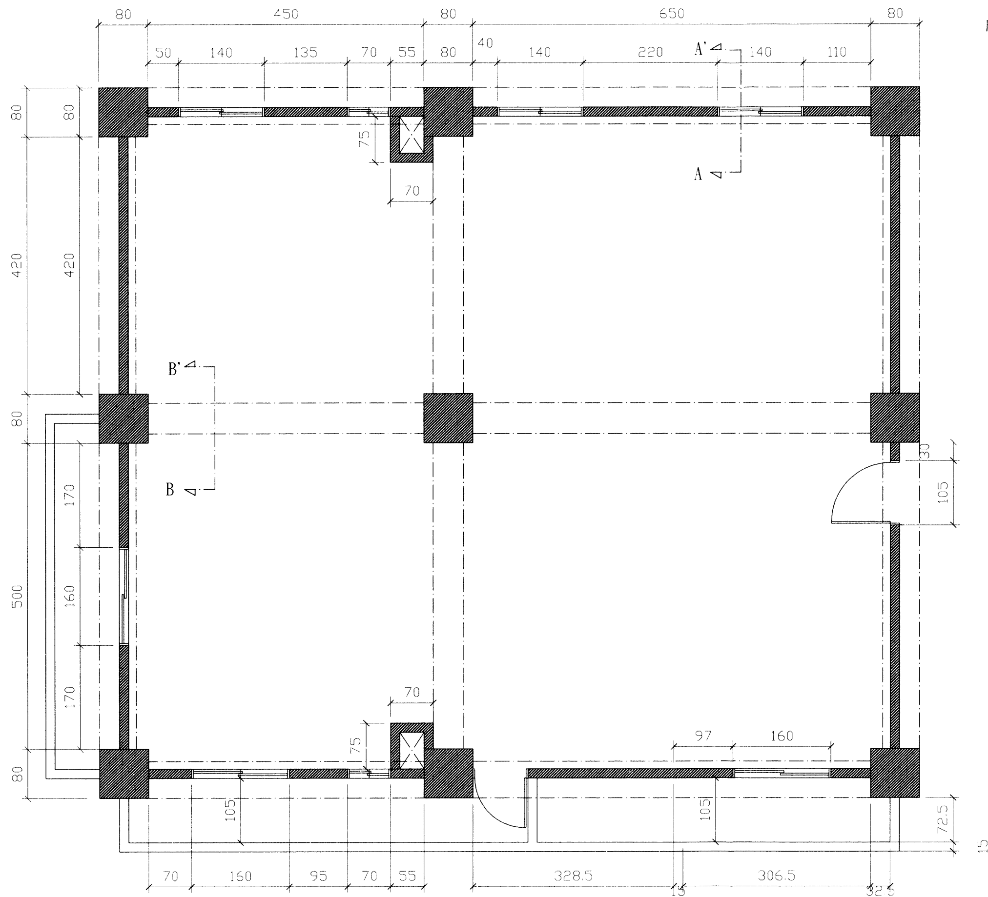
① 外樑處平面圖
