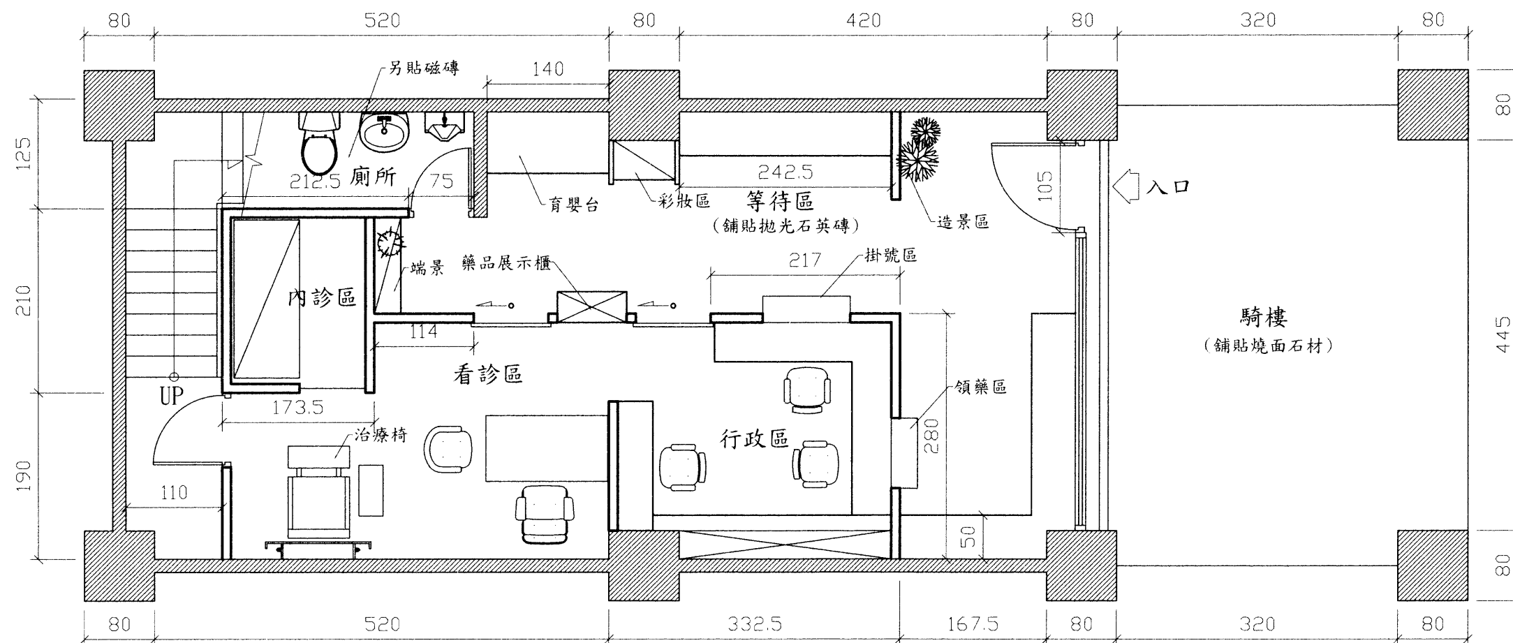
社區內科兒科診所 SCALE:1/60
