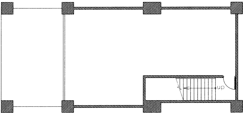
旅遊專業書籍專賣店原始平面圖
