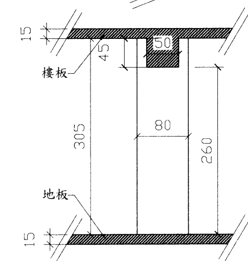
④ 中樑處剖面圖B-B'
