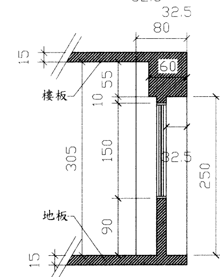
② 外牆處剖面圖A-A'
