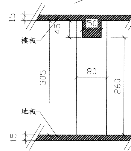
④ 中樑處剖面圖B-B'
