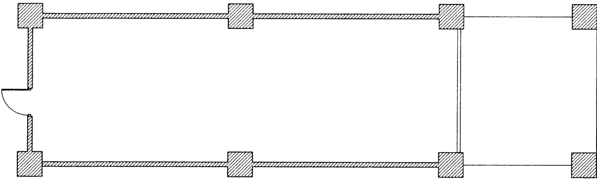
專業美容造型中心原始平面圖
