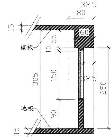
② 外牆處剖面圖A-A'
