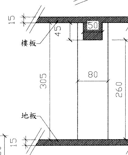
④ 中樑處剖面圖B-B'
