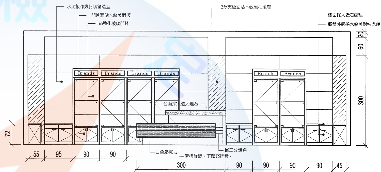
C向立面圖
