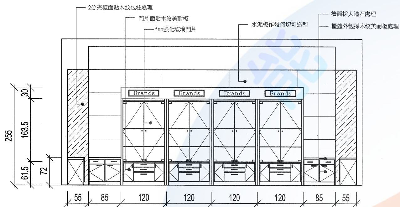
B向立面圖
