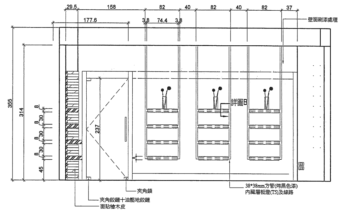
糕點販售區 D向 立面圖
