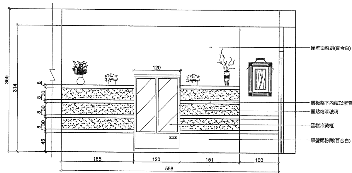
糕點販售區 C向 蛋糕冷藏櫃立面圖
