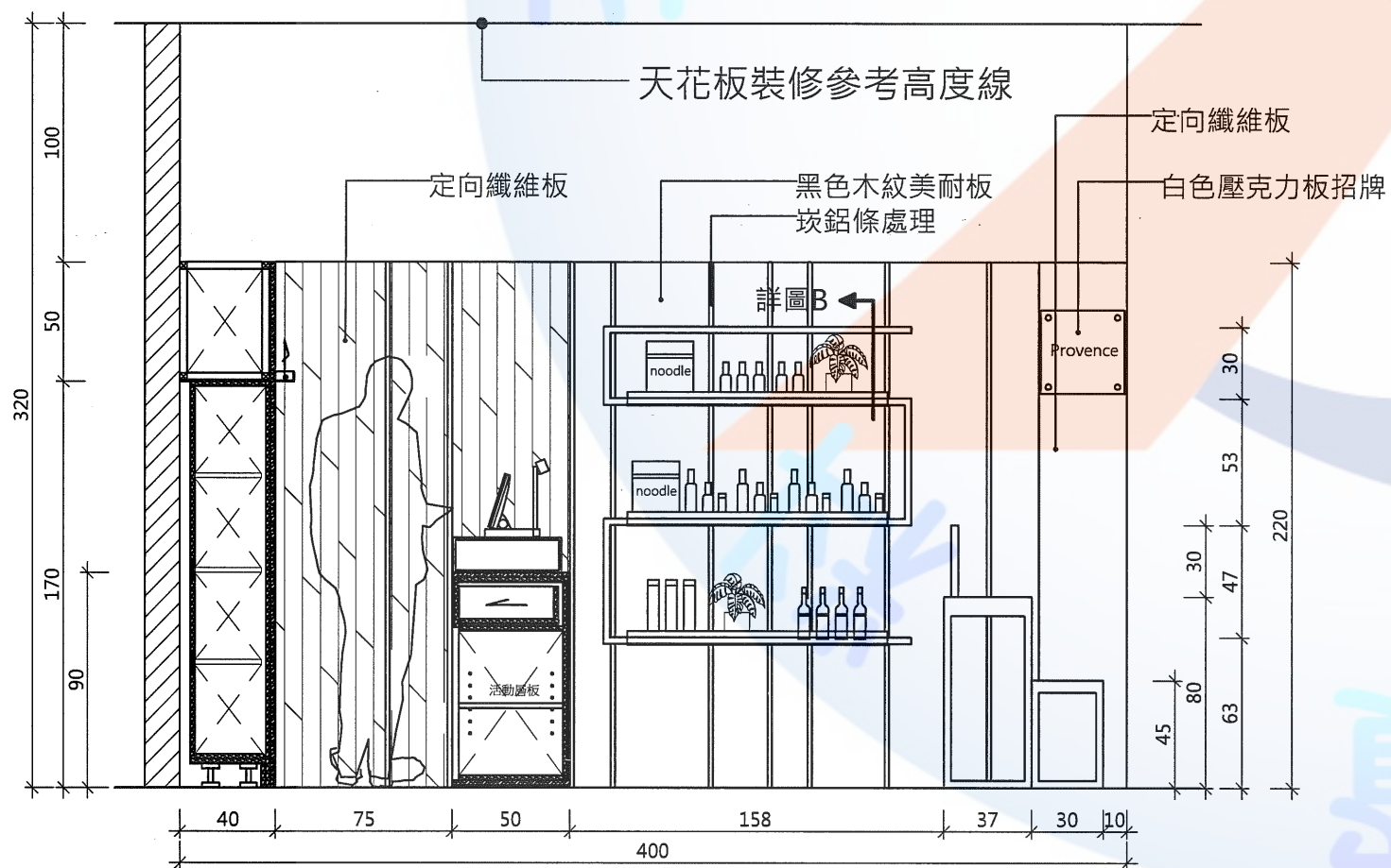
B向立面圖
