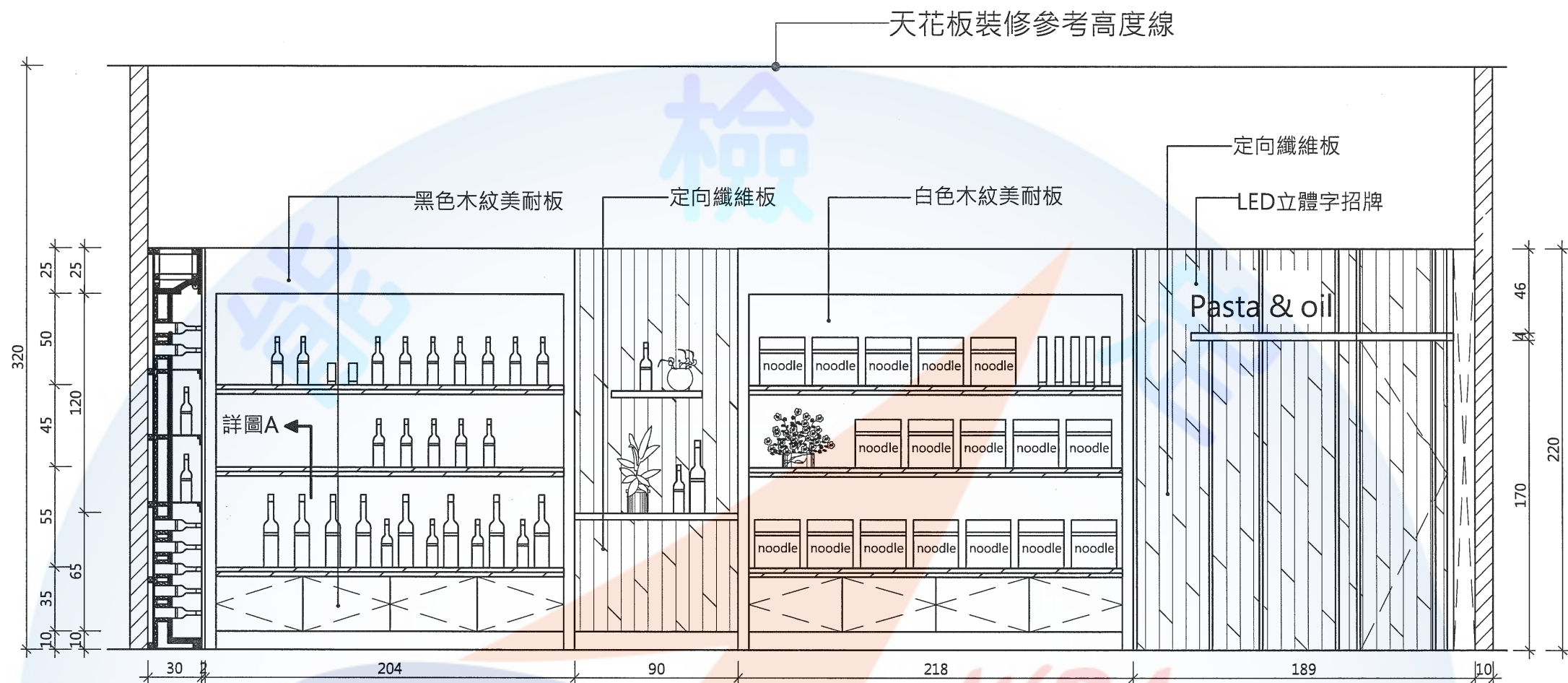
A向立面圖
