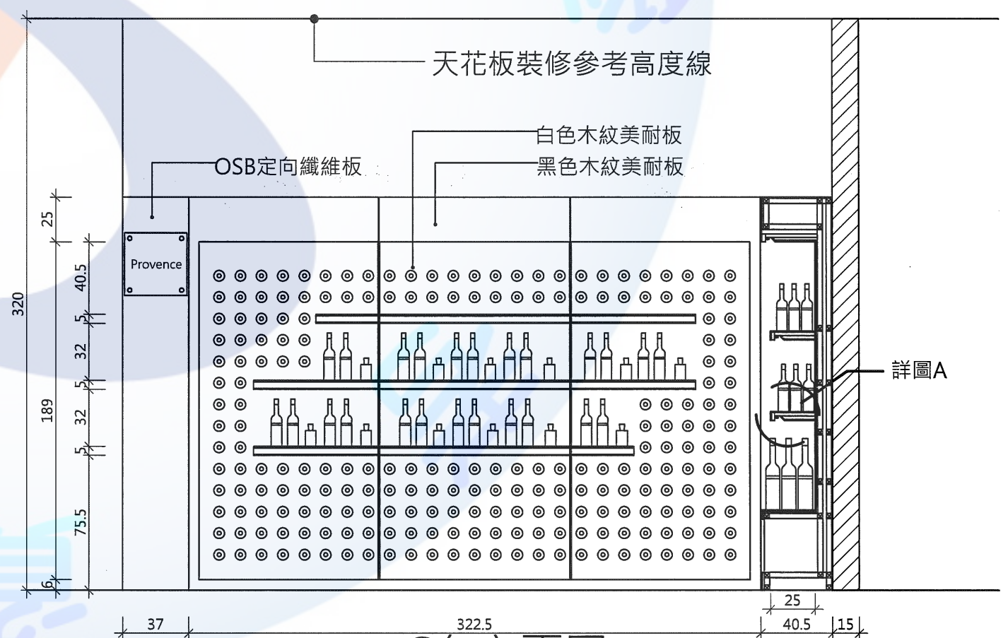
C向立面圖
