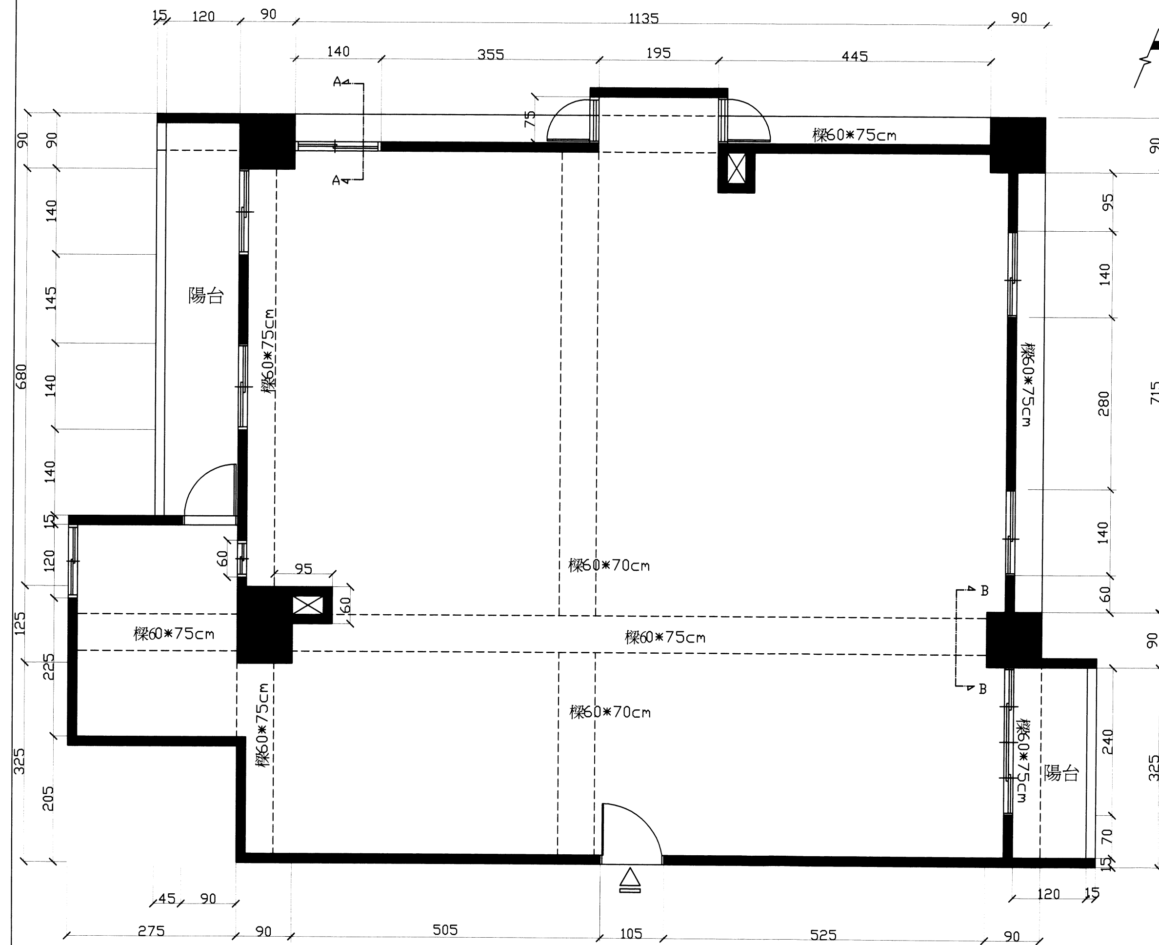
◎A-A平面圖
