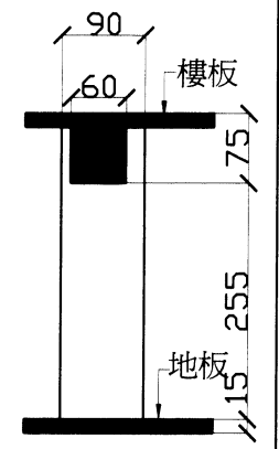
◎B-B剖面圖
