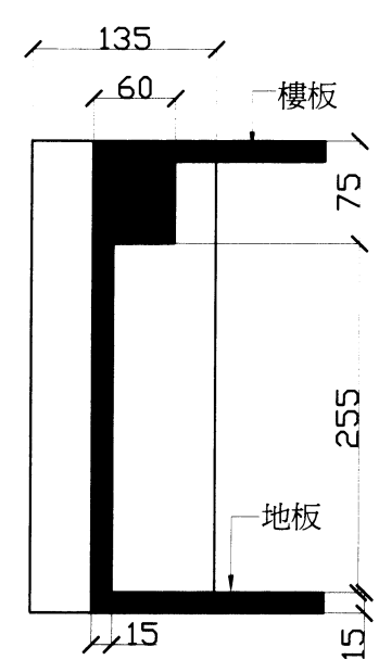
◎A-A剖面圖
