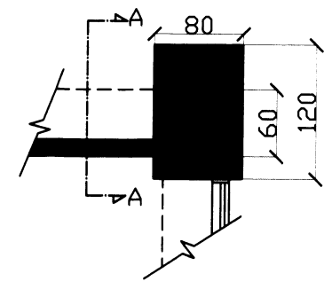
①A-A平面圖
