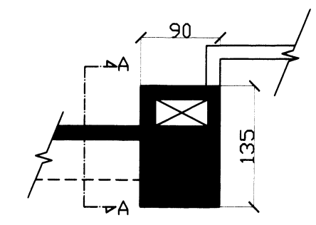
◎A-A平面圖
