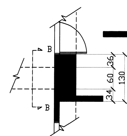
◎A-A平面圖
