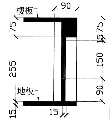
◎A-A剖面圖
