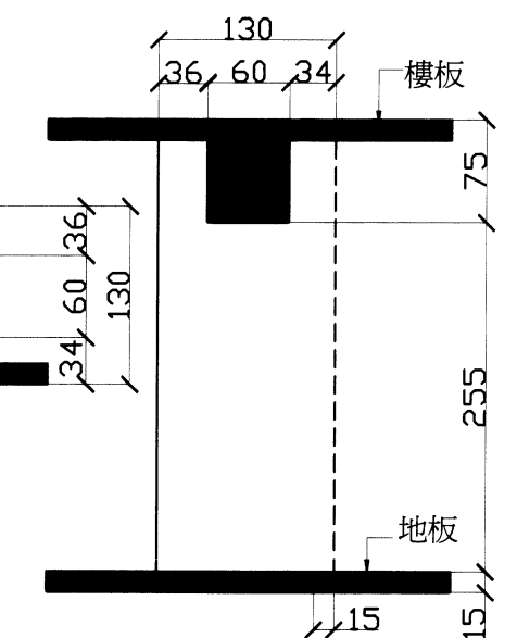
◎B-B剖面圖
