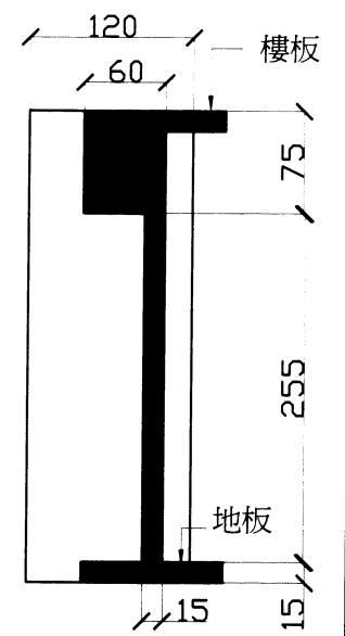
②A-A剖面圖
